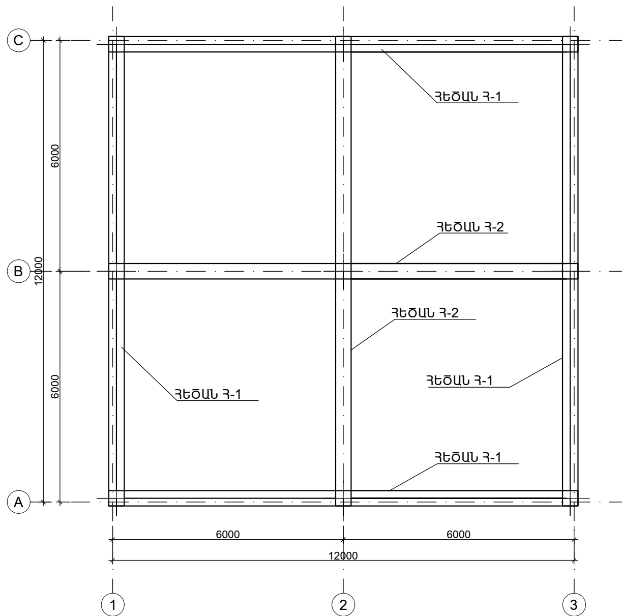
ՀԵԾԱՆՆԵՐԻ ՄԱԿՆԻՇԱՎՈՐՄԱՆ ՄԻՆԵՄԱ Մ1:100
