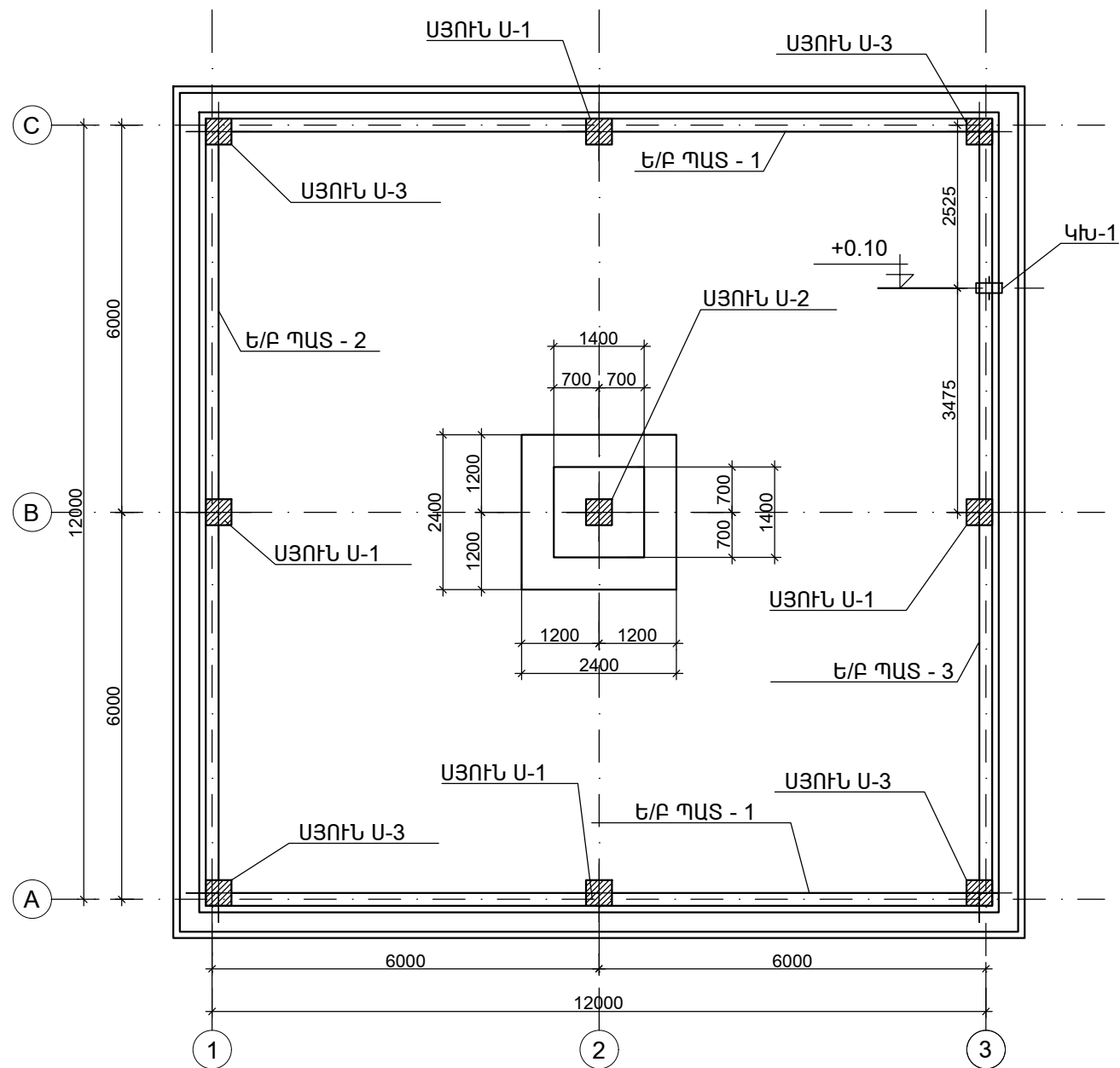
ՍՅՈՒՆԵՐԻ, Ե/Ք ՊԱՏԵՐԻ ՄԱԿՆԻՇԱՎՈՐՄԱՆ ՄԻՆԵՄԱ Մ1:100
