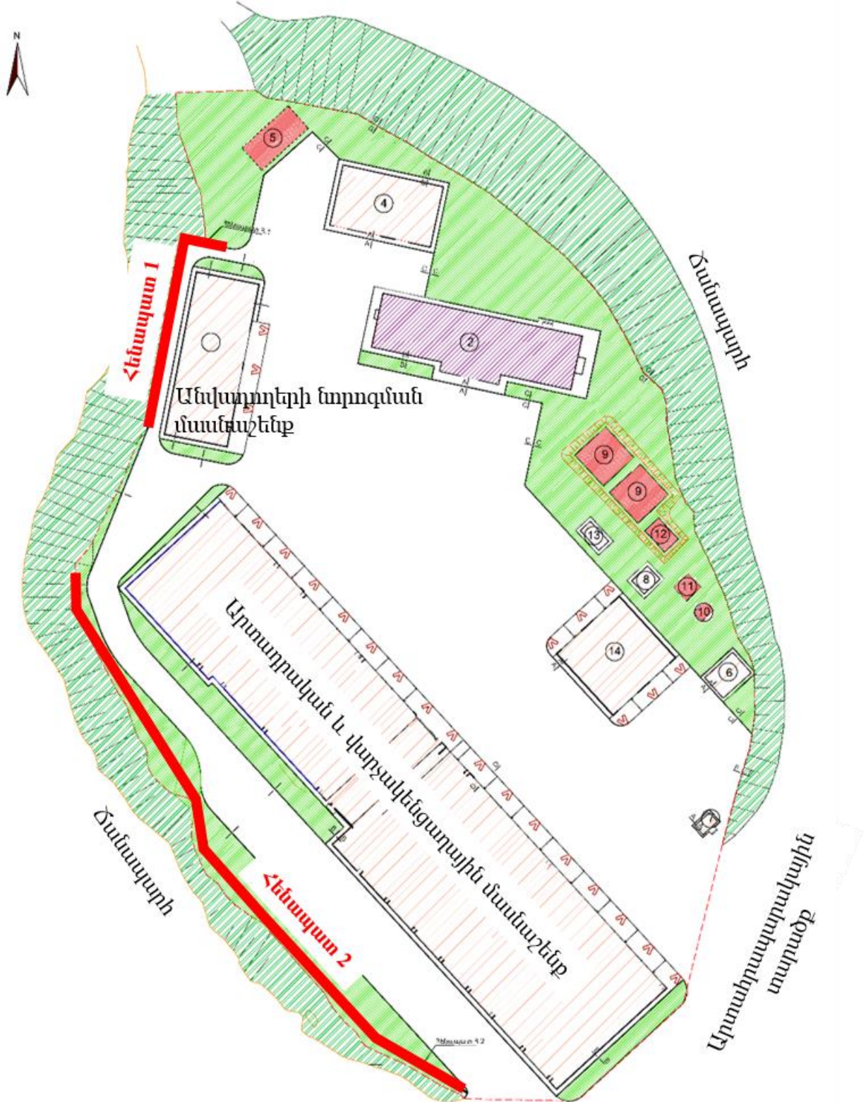
Նկ. 5.3. Գիզելային ավտոհավաքակայանի հատակագիծը՝ հենապատերի նշագրմամբ
