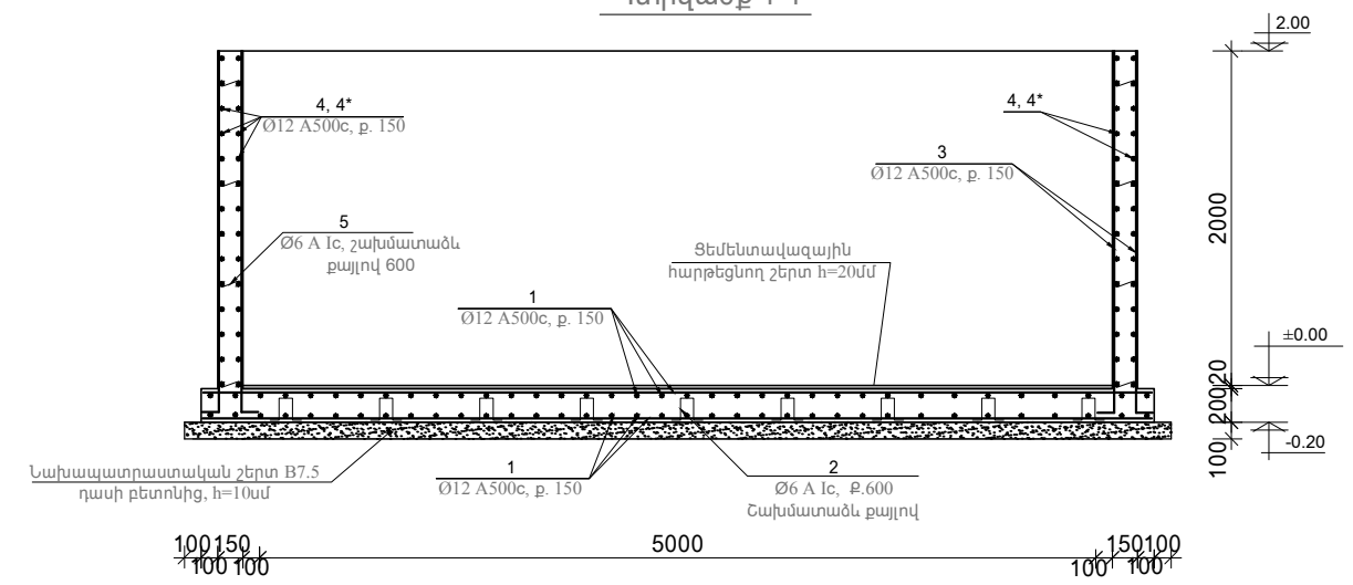
Կտրվածք 1-1
