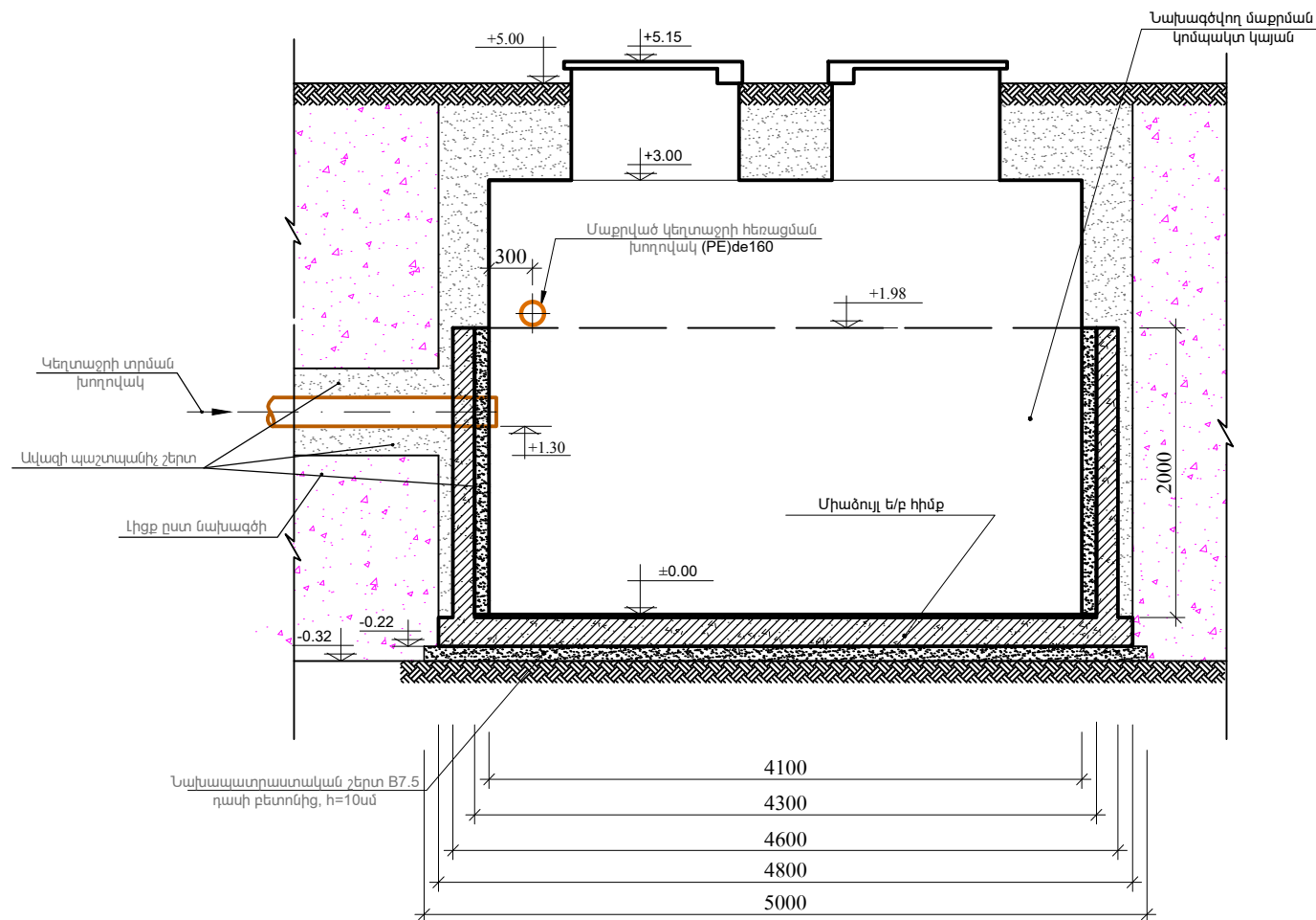
Կտրվածք 1-1
