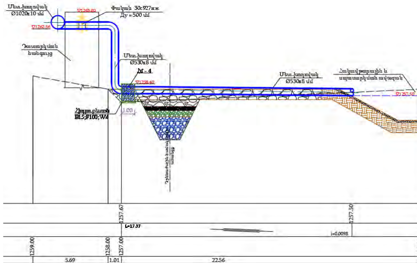
Նկ. 5.6. Դրենաժային համակարգի տիպային կտրվածք
