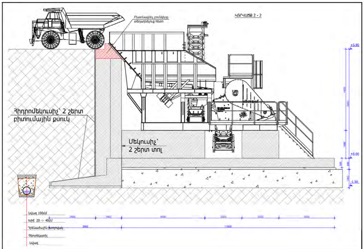
Նկար Զ3. 5. Ջարդիչ-տեսակավորող կայանի սխեման
