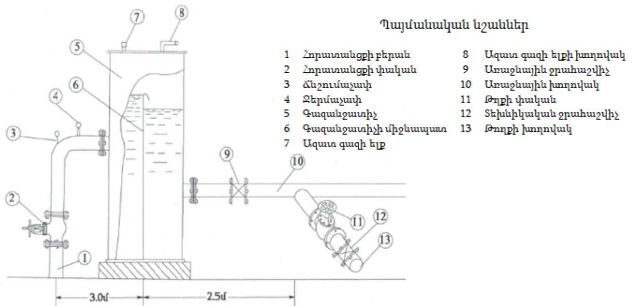
Նկ 19: Հանքային ջրի հորատանցքի գլխամասի սխեմա
