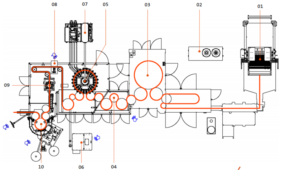
Նկ. 17: Kosme 3Bloc PET հոսքագծի նկարագիրը
