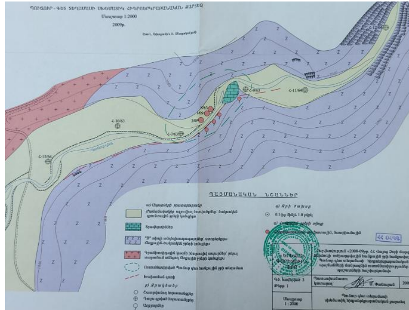
Նկ. 3: «Պուճուր գետ» տեղամասի սխեմատիկ հիդրոերկրաբանական քարտեզ
