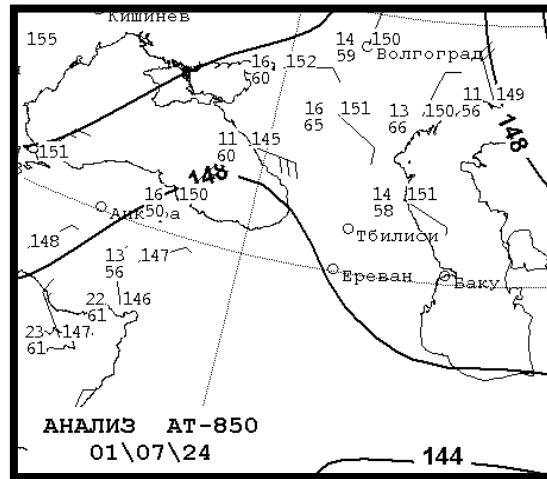
Նկար 38. Ճնշման դաշտը FS850մբ բարիկական քարտեզի վրա
