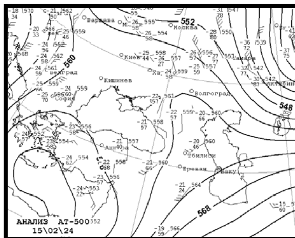
Նկար 14. Տաք ճակատը FS850մբ մակերևույթի քարտեզի վրա
