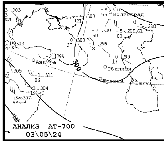
Նկար 21. Ճնշման դաշտը FS700-մբ բարիկական քարտեզի վրա
