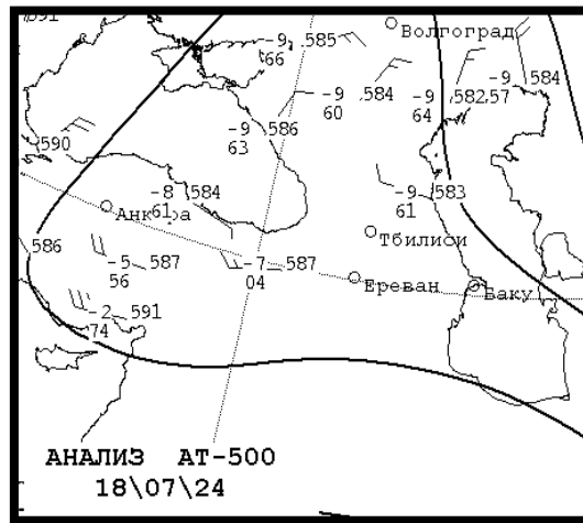
Նկար 47. Ճնշման դաշտը FS 500-ի բարիկական քարտեզի վրա
