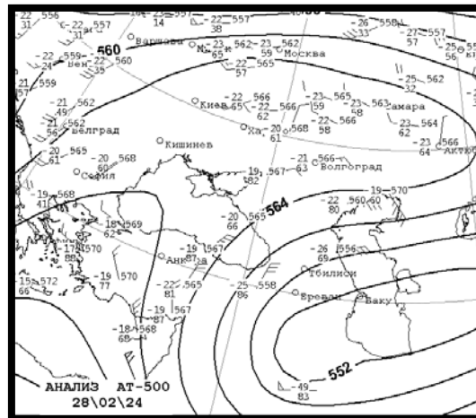
Նկար 18. Հյուսիս-արևելքից ներթափանցող արկտիկական ցուրտ օդային հոսանքները F500մբ մակերևույթի քարտեզի վրա
