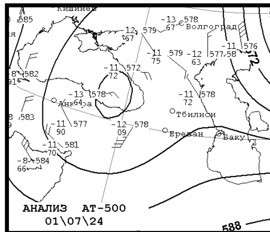
Նկար 39. Ճնշման դաշտը FS 500մբ բարիկական քարտեզի վրա
