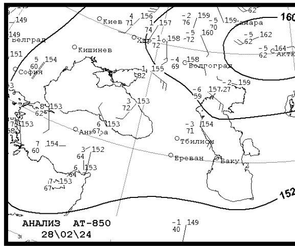
Նկար 17. Հյուսիս-արևելքից ներթափանցող արկտիկական ցուրտ օդային հոսանքները F850մբ մակերևույթի քարտեզի վրա
