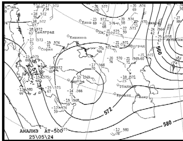
Նկար 34. Բարձր ցիկլոնը FS500-ի մակերևույթի վրա
