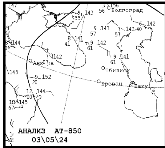
Նկար 20. Ճնշման դաշտը FS850-մբ բարիկական քարտեզի վրա
