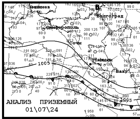
Նկար 37. Բարիկական դաշտերի դասավորությունը մթնոլորտի գետնամերձ շերտի սինոպտիկական քարտեզի վրա
