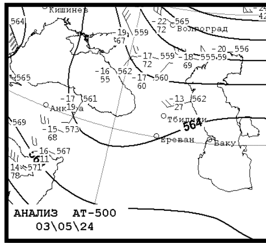
Նկար 22. Ճնշման դաշտը FS 500-ի բարիկազան քարտեզի վրա
