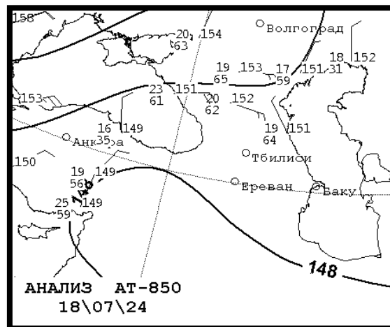
Նկար 46. Ճնշման դաշտը FS850մբ բարիկական քարտեզի վրա
