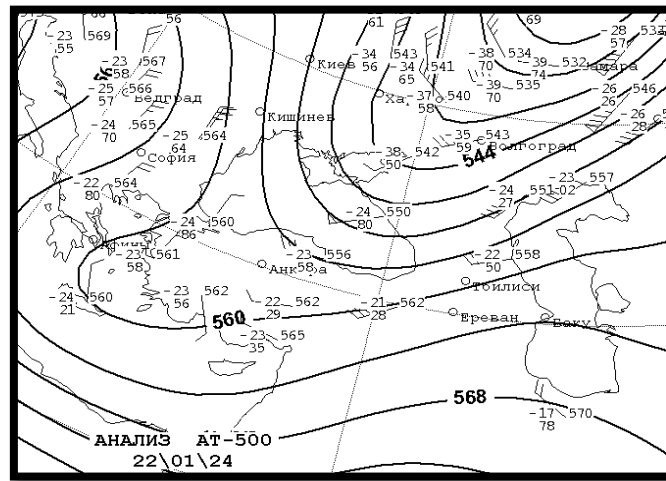
Նկար 6. Բարձր լաժքինան FS500մբ մակերևույթի քարտեզի վրա
