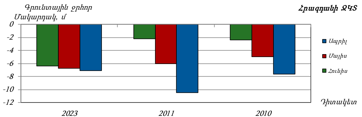
Գծապատկեր 70. Հրազդանի ՋԿՏ-ի գրունտային ջրերի մակարդակների փոփոխությունները
