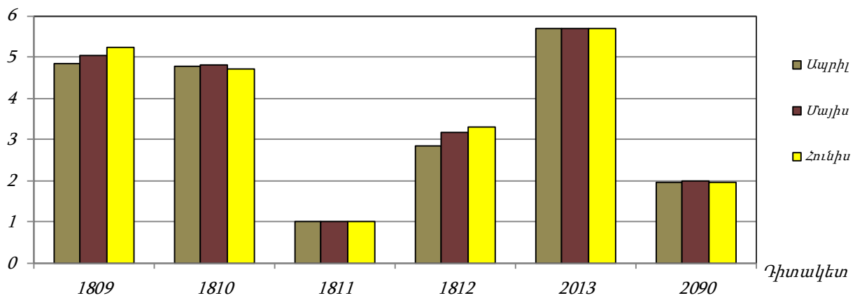
Գծապատկեր 77. Սևանի ՋԿՏ-ի շատրվանող հորատանցքերում մակարդակների փոփոխությունները
