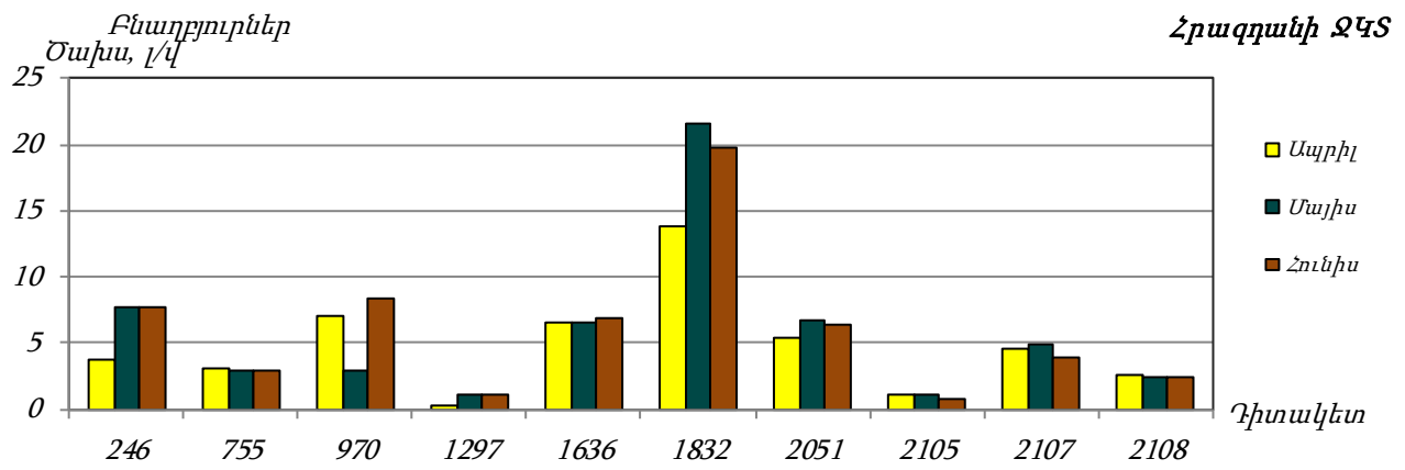
Գծապատկեր 65. Հրագրանի ՋԿՏ-ի բնադրյունների ծախսերի փոփոխությունները
