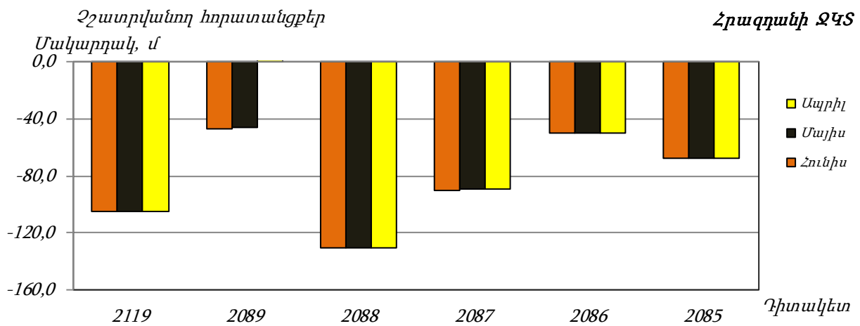
Գծապատկեր 69. Հրազդանի ՋԿՏ-ի չհատրվանող հորատանցքերի մակարդակների փոփոխությունները
