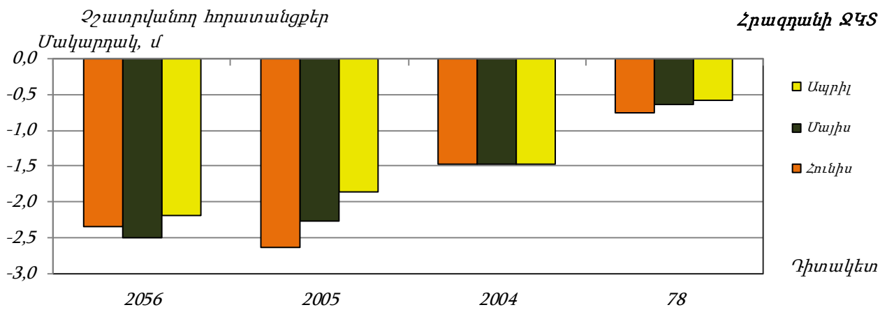
Գծապատկեր 68. Հրազդանի ՋԿՏ-ի չհատրվանող հորատանցքերի մակարդակների փոփոխությունները
