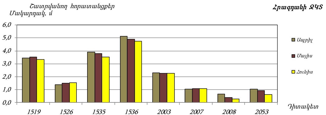
Գծապատկեր 67. Հրագրանի ՋԿՏ-ի շատրվանող հորատանցքերի մակարդակների փոփոխությունները
