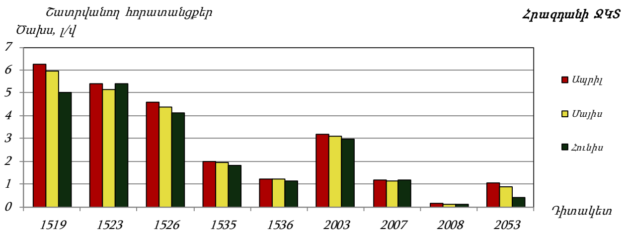
Գծապատկեր 66. Հրագրանի ՋԿՏ-ի շատրվանող հորատանցքերի ծախսերի փոփոխությունները
