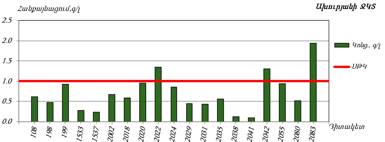
Փճապատկեր 60. Ախուրյանի ՋԿՏ-ի դիտակետերում հանքայնացման պարունակությունը
