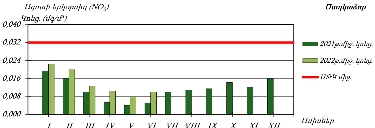
Գծապատկեր 45. Ծաղկաձոր քաղաքի մթնոլորտային օդում ազոտի երկօքսիդի միջին ամսական կոնցենտրացիաների փոփոխությունները
