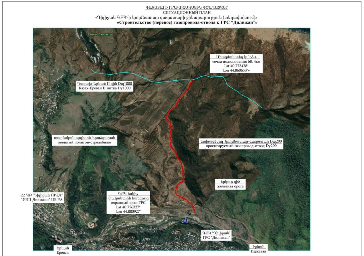
Նկար 2. Գազատարի իրավիճակային սխեման
