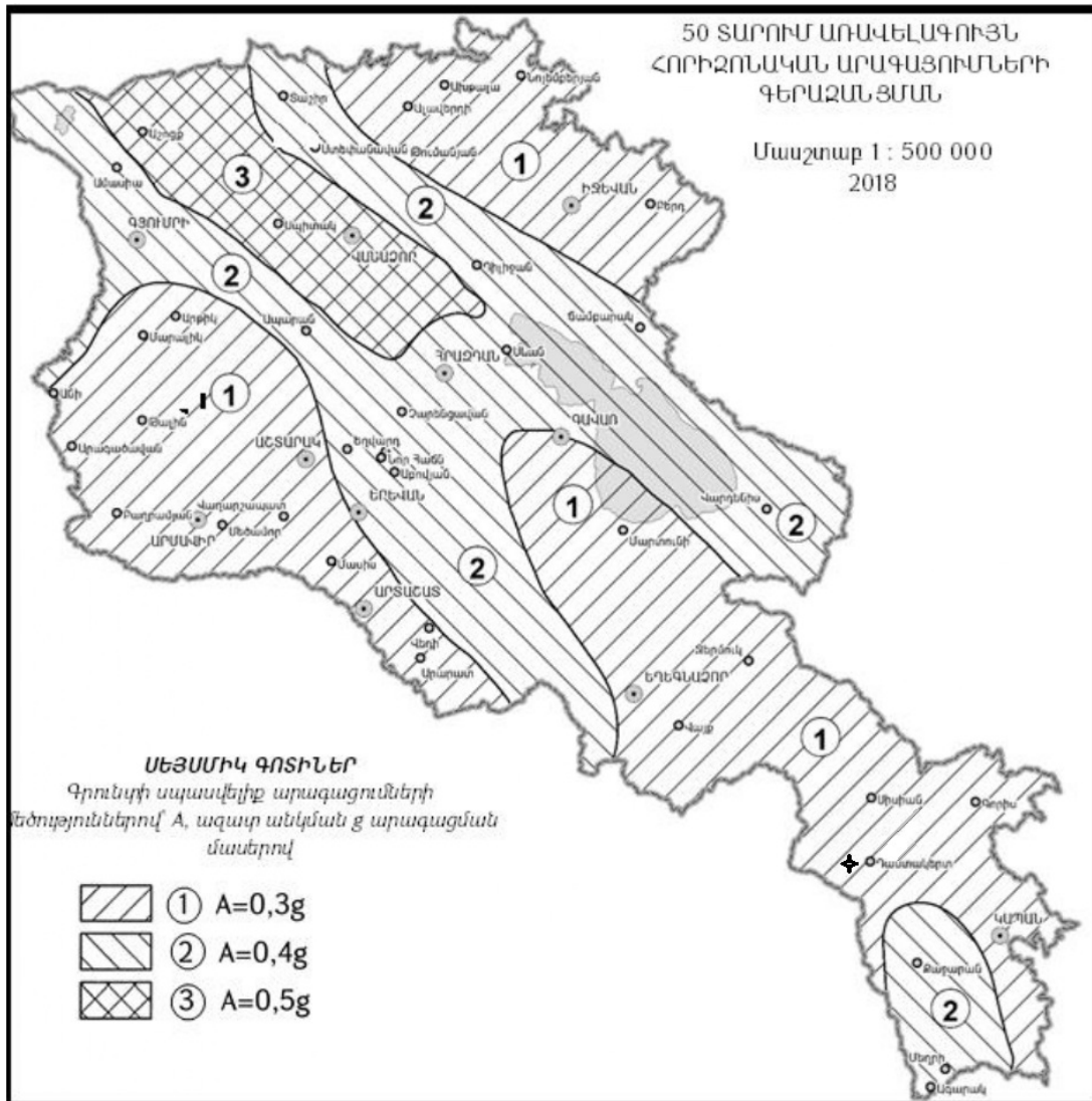
Նկ. 5: ՀՀ տարածքի հավանական սեյսմիկ վտանգի գոտիավորման քարտեզ, ըստ է ՀՀՇՆ 20.04- «Երկրաշարժադիմացկուն շինարարություն. նախագծման նորմեր» հավելանախ 1 -ի:
