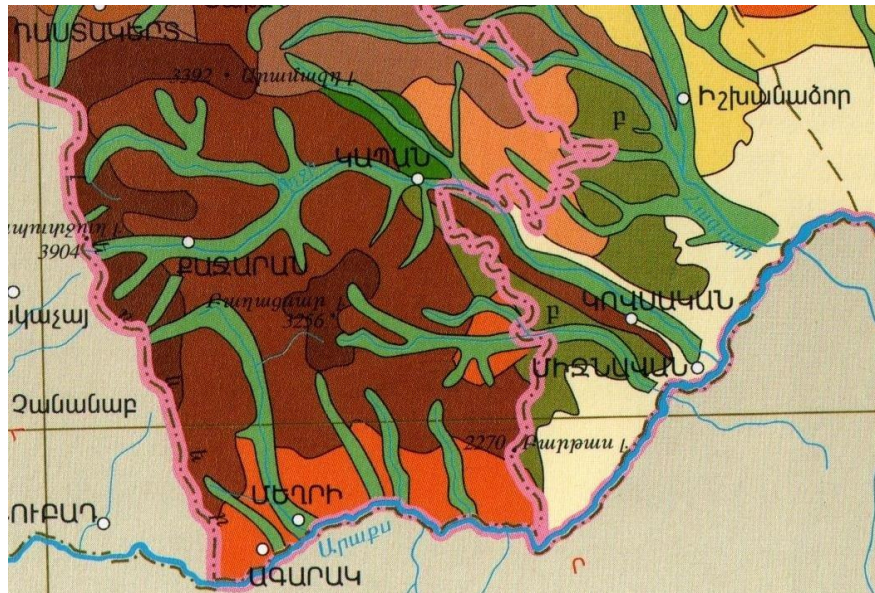
Նկար 4. Երկրաձևաբանություն
