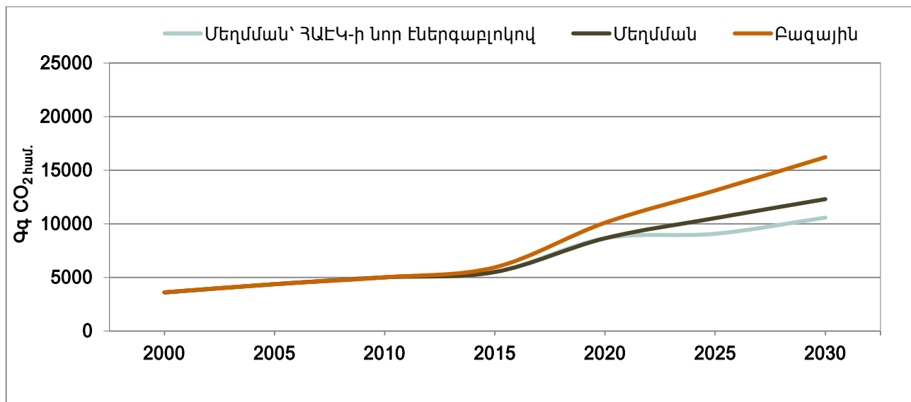
Նկար 4-2. Ջերմոցային գազերի արտանետումներն «Էներգետիկա» սեկտորում 2000-2010թթ. և կանխատեսումը մինչև 2030թ.
