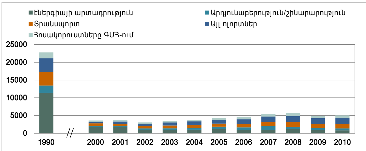
Նկար 2-7. Ջերմոցային գազերի արտանետումները «Էներգետիկա» սեկտորում, 1990-2010թթ.
