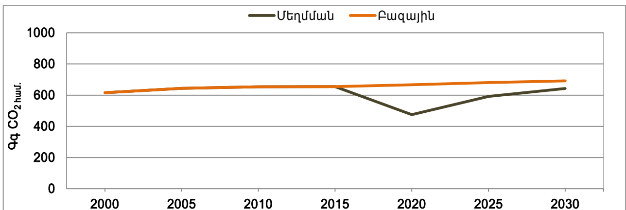
Նկար 4-6. Ջերմոցային գազերի արտանետումները 2000-2010թթ. և կանխատեսումը մինչև 2030թ. «Թափոններ» սեկտորում
