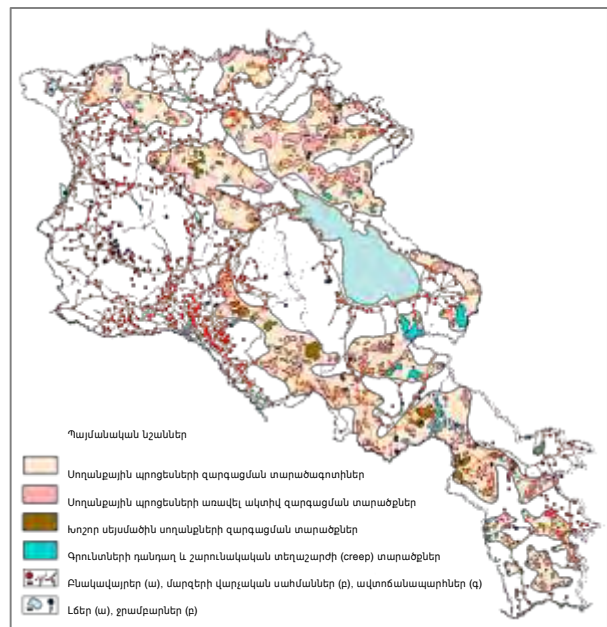
Նկար 5-12. Հայաստանի բնակավայրերի և ենթակառուցվածքների տարածական տեղադիրքը սողանքավտանգ գոտիների նկատմամբ
