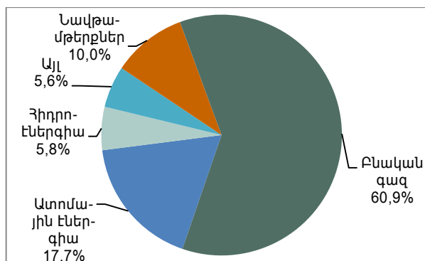
Սկար 1-3. Հայաստանում Էներգիայի աղբյուրների մասնաբաժինն ընդհանուր Էներգասպառման մեջ, 2012թ.
