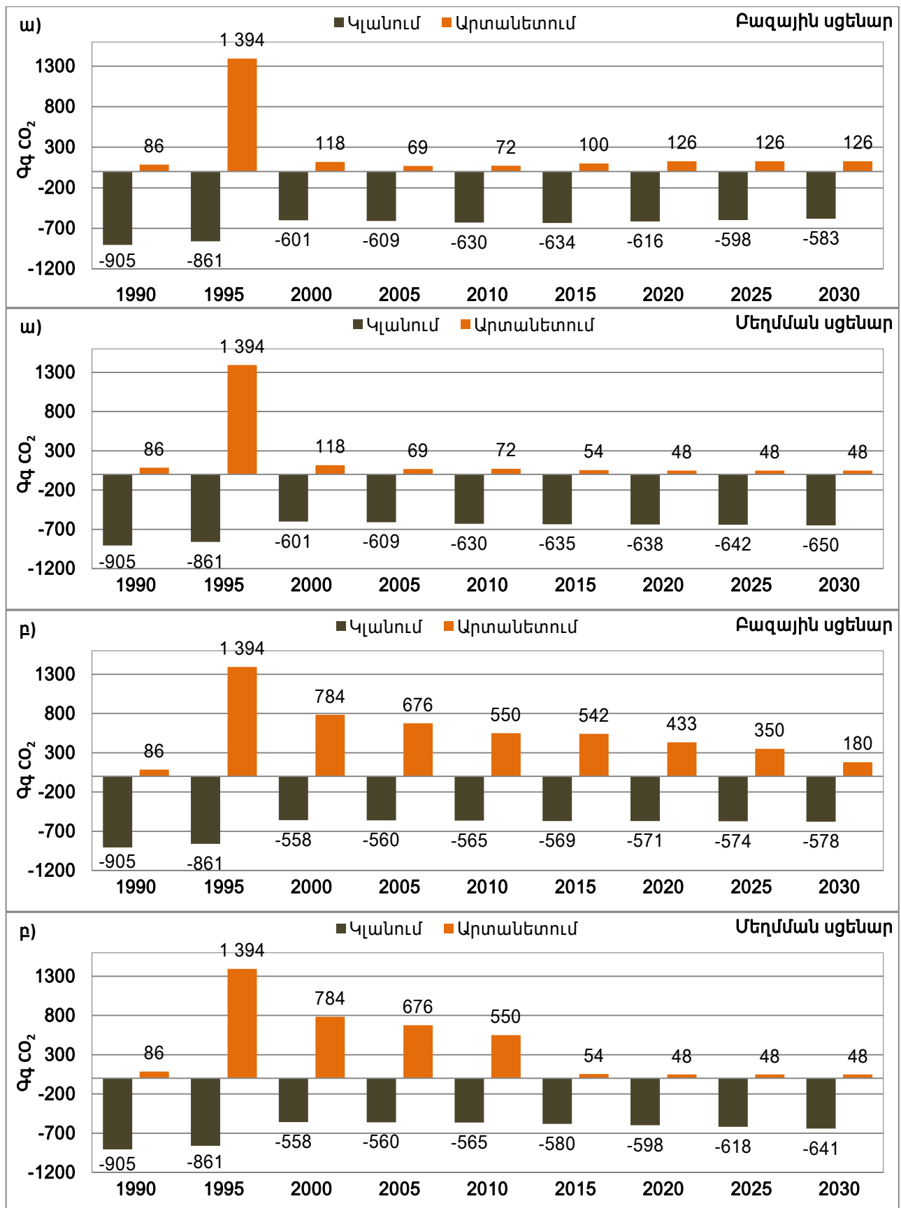
Նկար 4-5. Հայաստանի անտառներում CO 2 -ի կլանումները/արտանետումները 1990-2010թթ. և կանխատեսումը մինչև 2030թ. (ա) 2000-2010թթ. ըստ պաշտոնական տվյալների, (բ) ըստ փորձագիտական գնահատականի:
