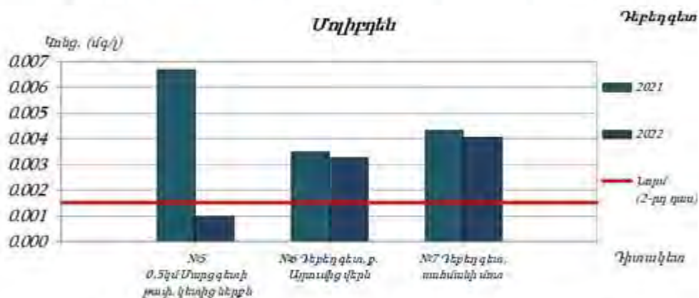
Գծապատկեր 5. Դեբեդ գետում մոլիբդենի կոնցենտրացիայի փոփոխությունը
