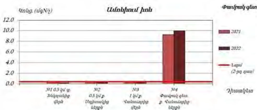
Գծապատկեր 4. Փամբակ գետում ամոնիում իոնի կոնցենտրացիայի փոփոխությունը
